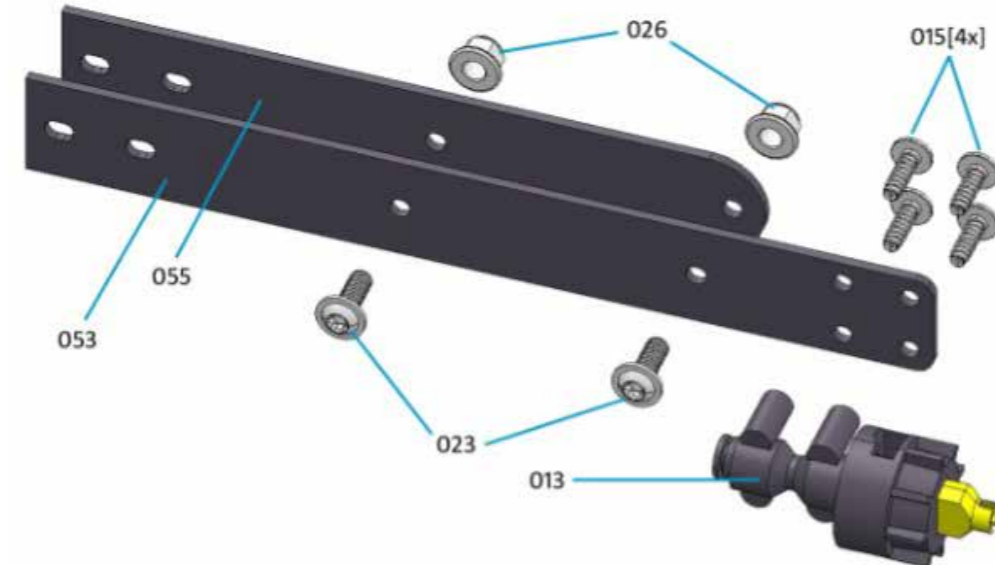
Voorbeeld samenstelling dopbevestiging enkel dophouder
