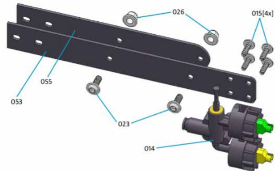
Voorbeeld samenstelling schuif-dophouder
