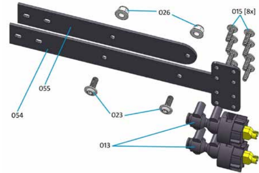
Voorbeeld samenstelling twee enkele dophouders
