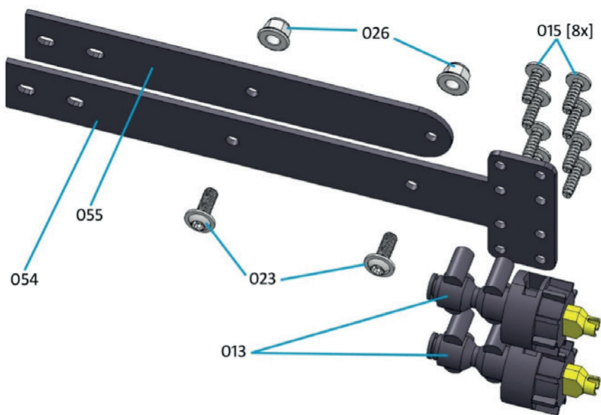
Voorbeeld samenstelling twee enkele dophouders
