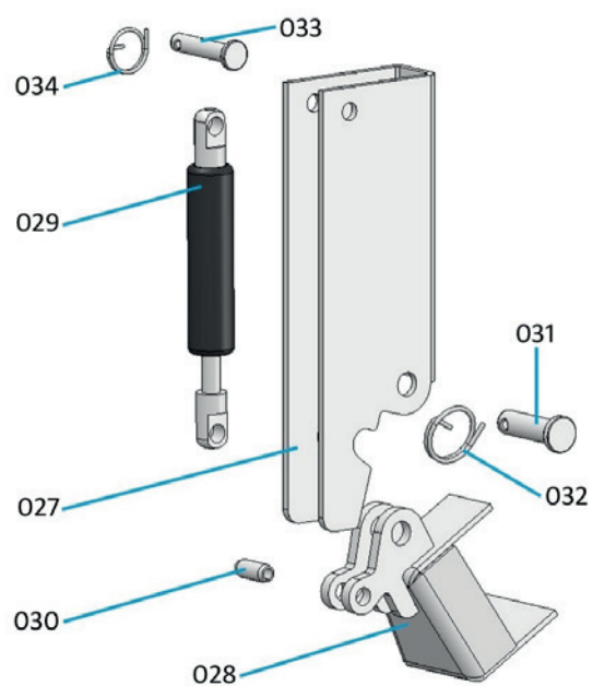
Voorbeeld samenstelling gepatenteerde Wingophanging
